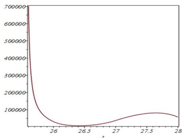
شکل ۵. مشتق شاخص کل نسبت به قیمت نفت سبد اوپک در بازه از اواسط ماه ۲۵ تا ماه ۲۸
