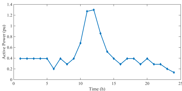
شکل ۱۱. منحنی روزانه توان اکتیو مجموع سیستم‌های بادی
