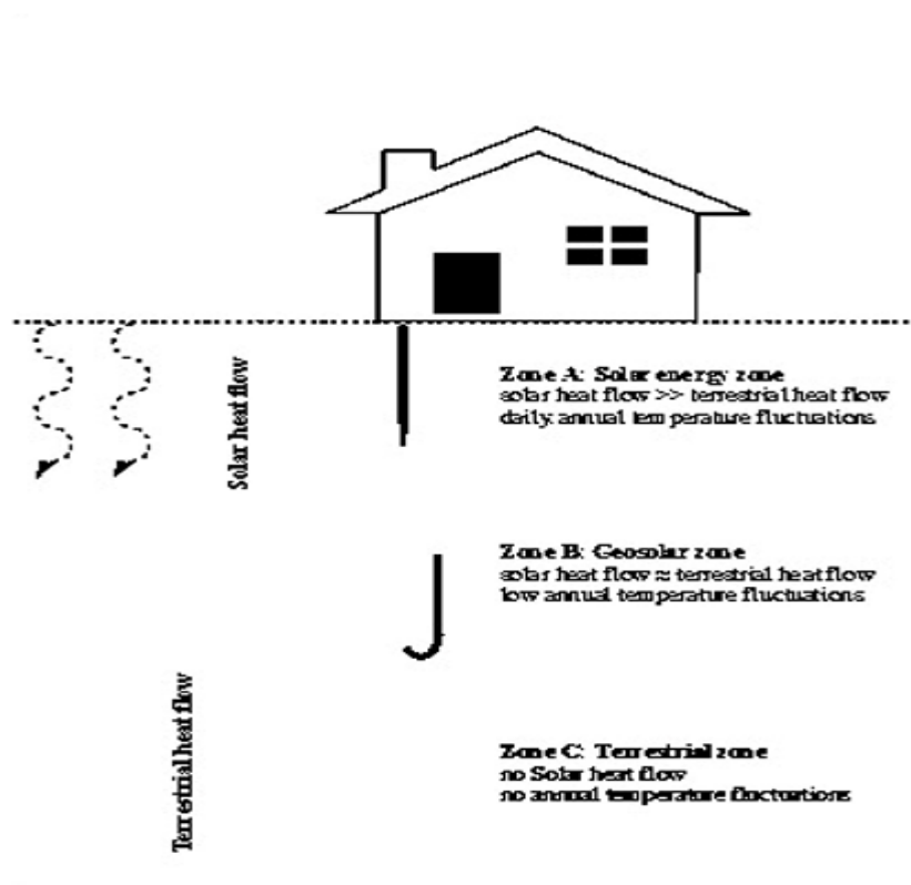
شکل ۱- دسته‌بندی نواحی زمین‌گرمایی بر حسب شار حرارتی تابش‌های خورشید و شار حرارتی درون زمین [۳]
